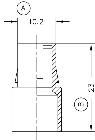
Secc. C-C'
