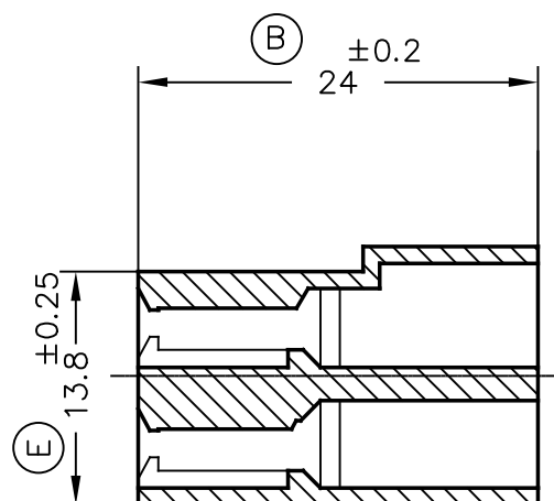
Secc. B-B'
