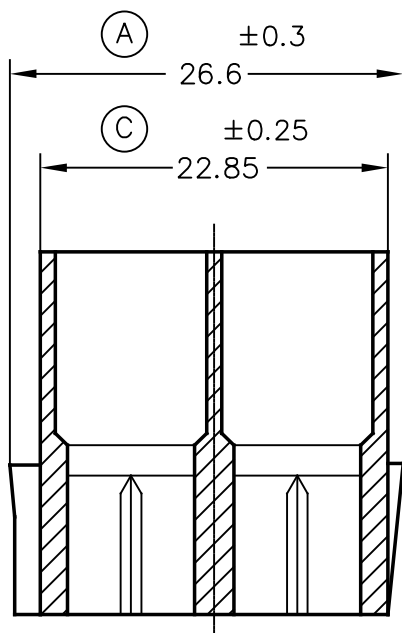
Secc. A-A'
