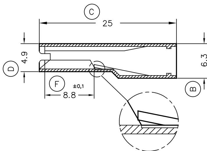
Secc. B-B'
