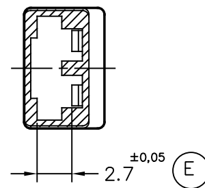
Secc. A-A'
